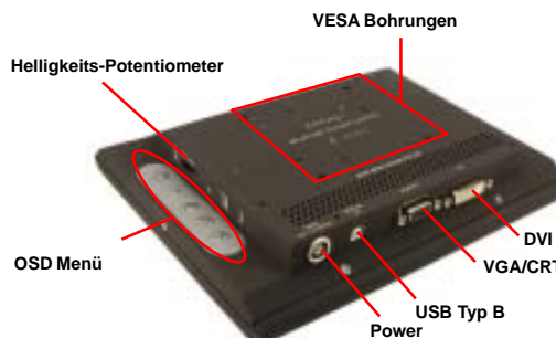
Rücksansicht DeltaVarioMon 6,5" ^
