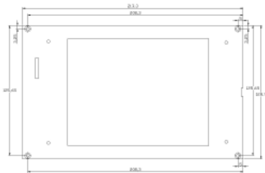
Frontansicht
