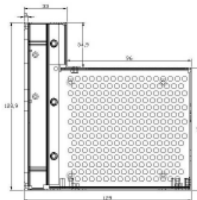
Seitenansicht
