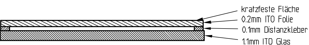
Schnitt A-A
